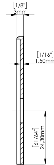
SEZIONE A-A
